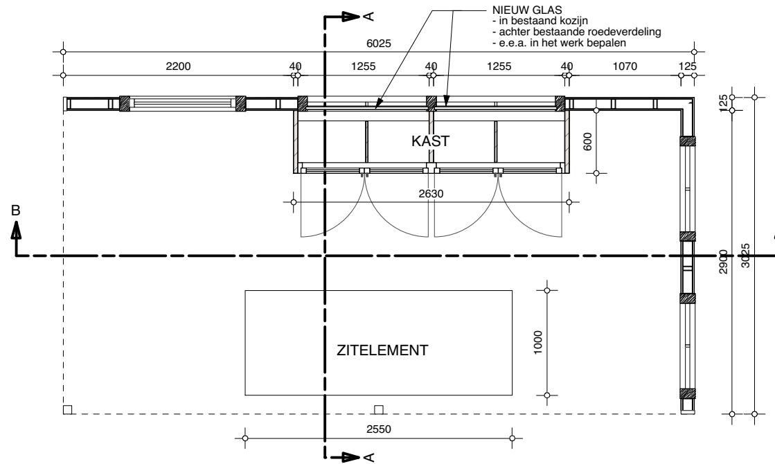
PLATTEGROND
