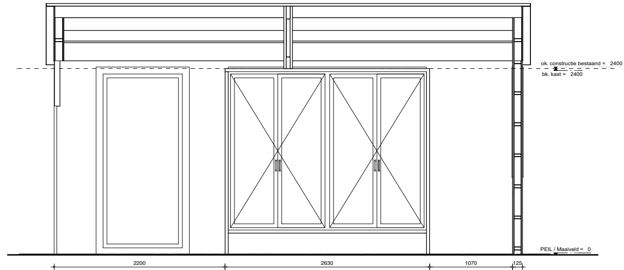
DOORSNEDE B-B
