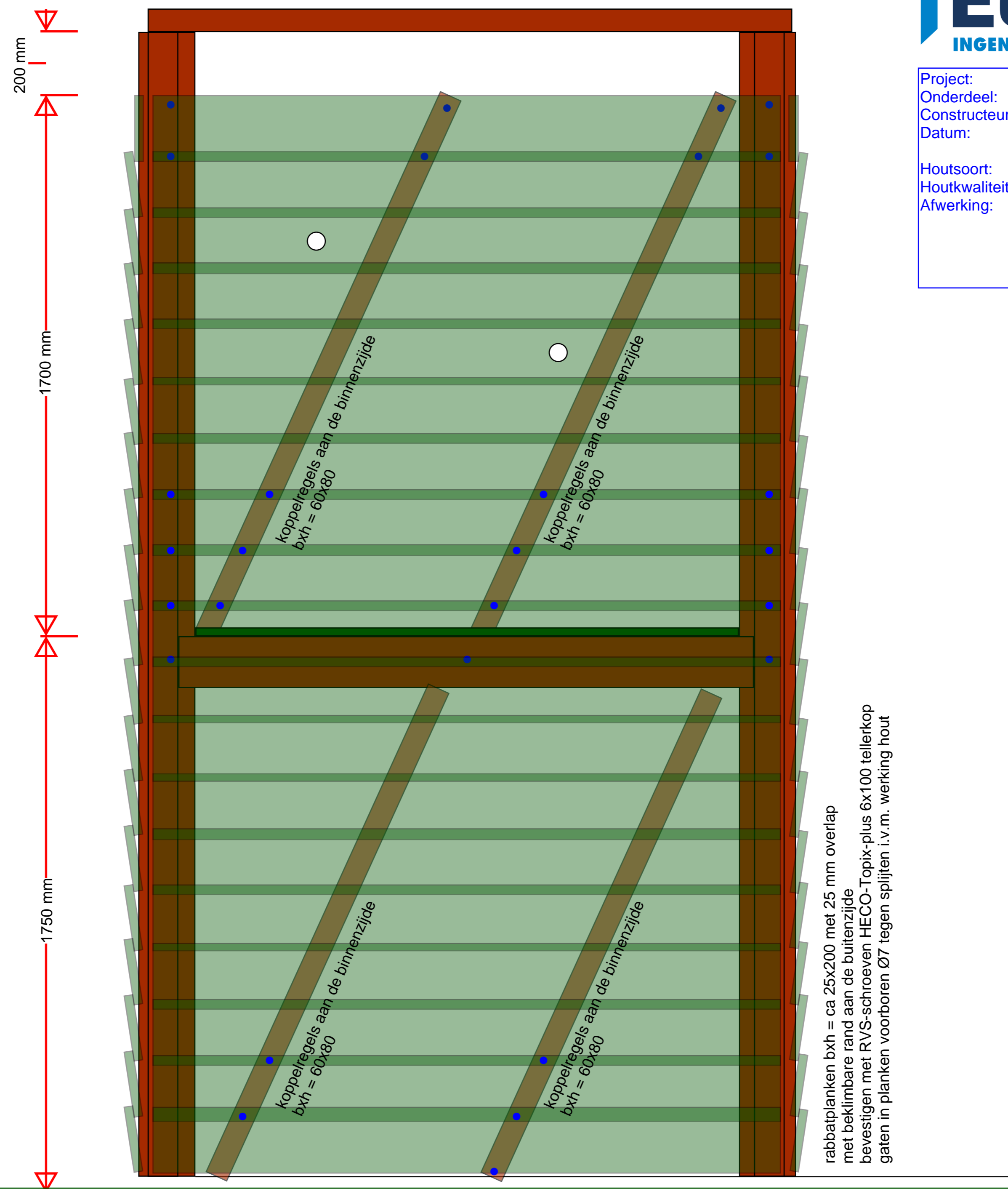
AANZICHT DICHTE ZIJDE
