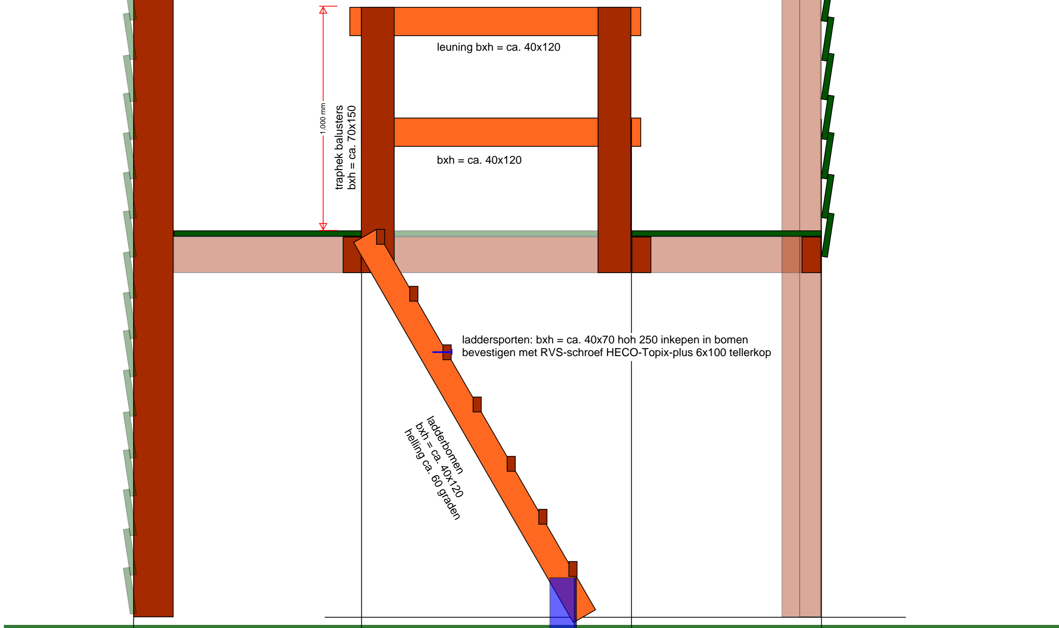
DOORSNEDE TRAPGAT MET LADDER
